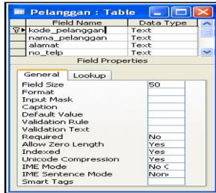
Contoh data tabel pelanggan :
