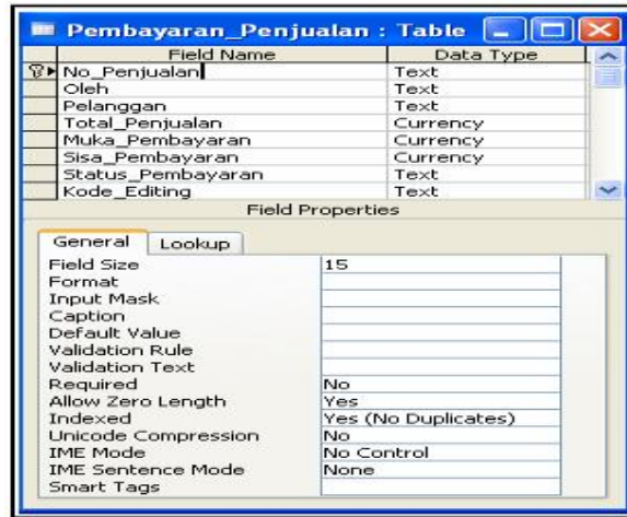
Contoh data tabel pembayaran penjualan :
