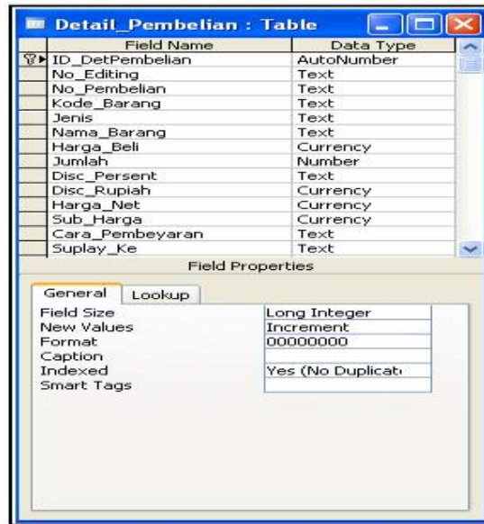
Contoh data tabel detail pembelian :
