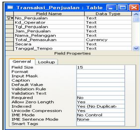
Contoh data tabel transaksi penjualan :
