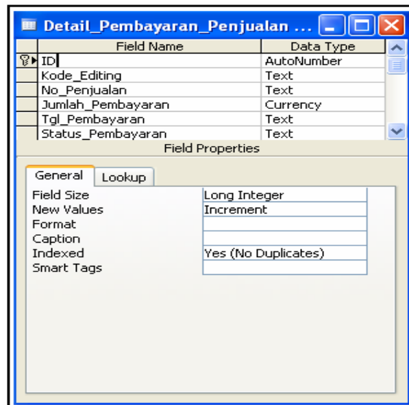
Contoh data tabel detail pembayaran penjualan :
