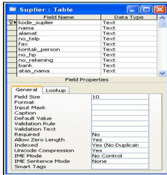
Contoh data tabel suplier :
